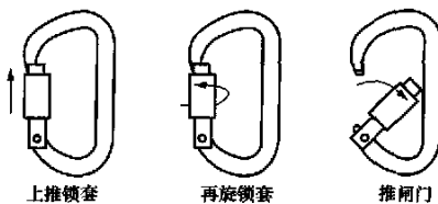
c) 推旋型自锁连接器
