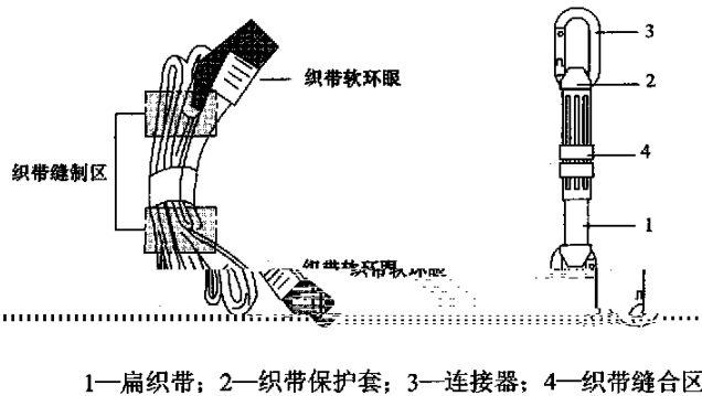
图 5 织带型缓冲器典型结构和主要部件示意图
