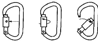
b) 压旋型自锁连接器
