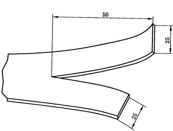
图 10 抗撕裂试验试品尺寸
