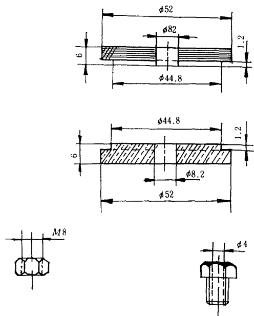
图 A4 保护电极(A)(B)部件结构
